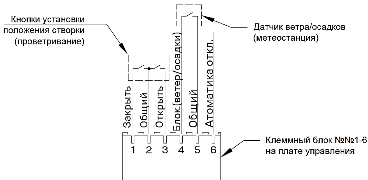
Рис. 7. Схема подключения кнопок установки положения (продветривания) и датчиков ветра/осадков (метеостанции)
