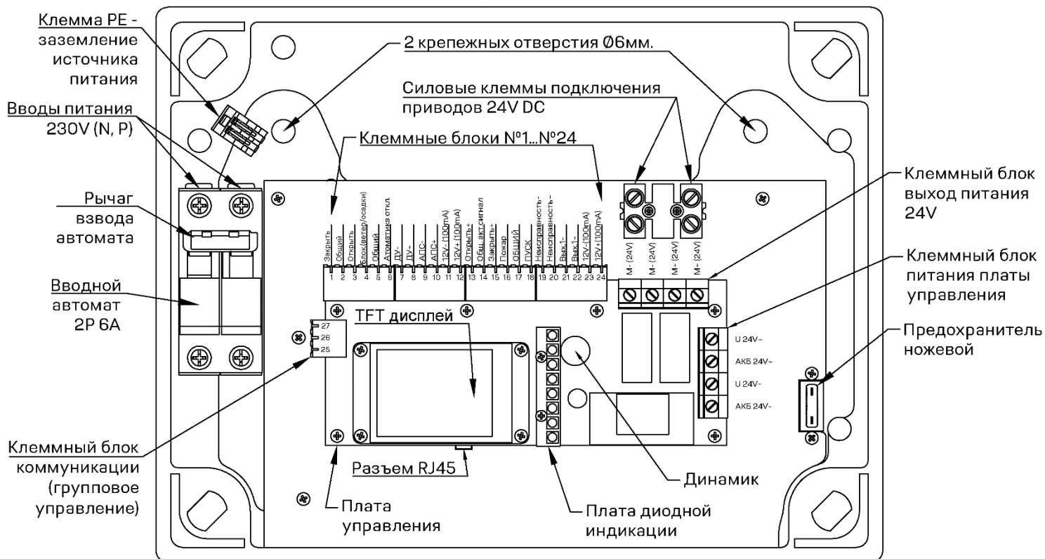
Рис. 2. Органы управления NRD-01 2420DC (20A)
